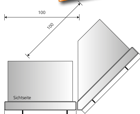
Zweiteilige 135° Innenecken werden aus einem Element der 90° Innenecke und einem Standardelement. Innenecke Sichtbeton INNEN 100/100 cm zweiteilig 135°
